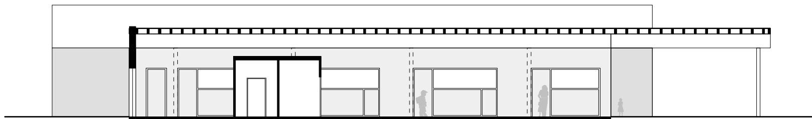
Langse snede BB'
