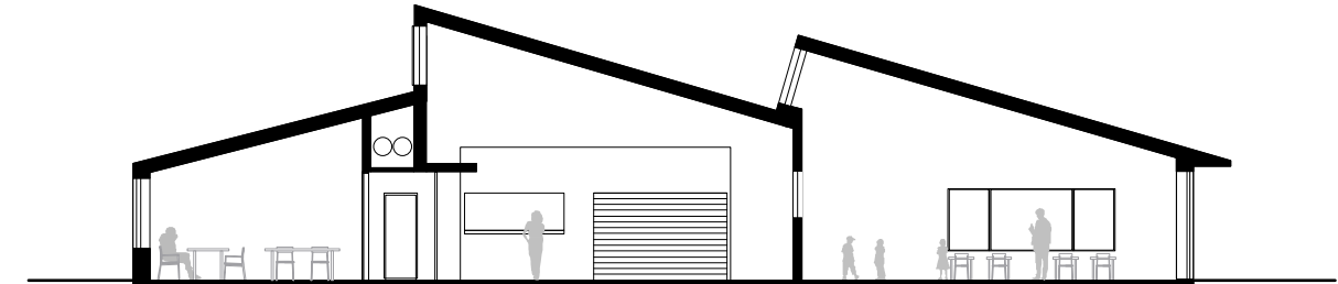
Dwarse snede CC'
