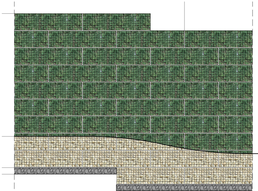
VULMATERIAAL: combinatie geotextiel en teelaarde, gestuurde of spontane begroeiing
