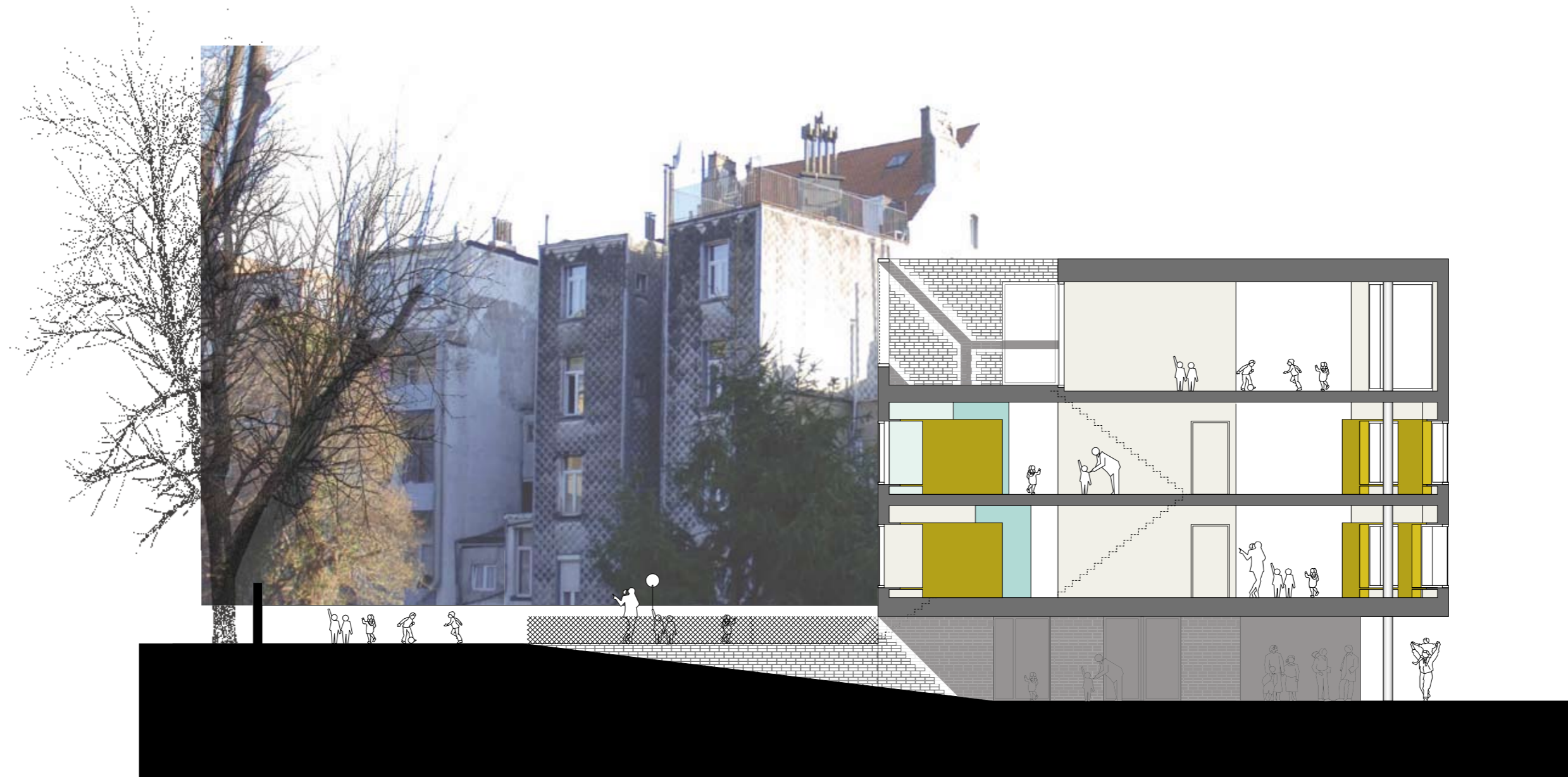
LANGSSNEDE B-B
